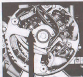
Figura D – Cercare l'alloggio delle spazzole di carbone. E' possibile sostituire questo elemento in caso di sua usura eccessiva
