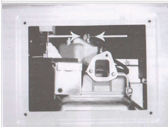
Figura A – Rimuovere il pannello laterale, poi togliere il filtro d'aria. Cercare la leva di decompressione „rossa” (nell'immagine di cui sopra si trova sulla posizione SU (UP)). Premere la leva di decompressione verso il basso—questa cosa porterà all'apertura della valvola di scarico. Riposizionare al suo posto il gruppo con filtro d'aria. Accendere il motore. Si può osservare che la leva a molla ritornerà automaticamente sulla posizione SU (UP). (Denominato anche gruppo di decompressione su alcuni schemi.)
