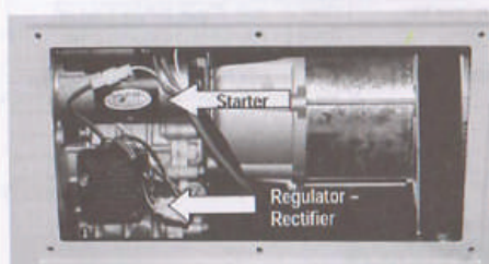
Figura C – Cercare l'alloggio del pannello di accesso posteriore, che è stato rimosso. Si può vedere l'alloggio dell'avvitatore e del regolatore / raddrizzatore per la batteria di avviamento da 12V. Il motore dell'avvitatore si trova al di sopra del regolatore/raddrizzatore.
