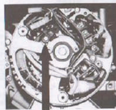
Figura D – Căutați locația perilor de cărbune. Este posibil ca acest element să trebuiască să fie schimbat când se uzează excesiv.
